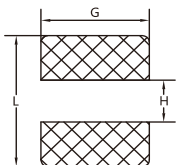
焊盘尺寸/Pad size
