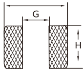
焊盘尺寸/Pad size
