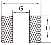
焊盘尺寸/Pad size
